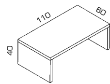
Couchtisch Bestell-Nr. 830-20 D2
