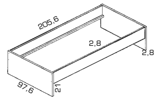
EB 1 90 x 190 cm Nr. 830700 90 x 200 cm Nr. 830701 90 x 210 cm Nr. 830702 100 x 200 cm Nr. 830703
