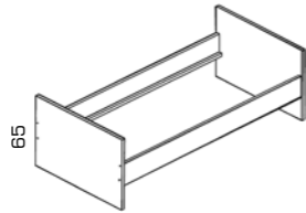
EB 2 90 x 190 cm Nr. 830720 90 x 200 cm Nr. 830721 90 x 210 cm Nr. 830722 100 x 200 cm Nr. 830723
